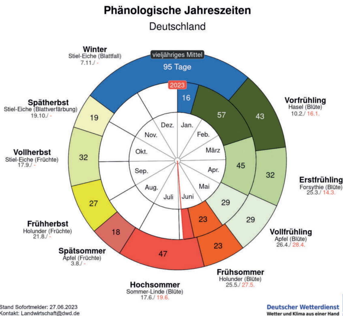
Abb. 4: Phänologische Uhr. Quelle: Deutscher Wetterdienst.
